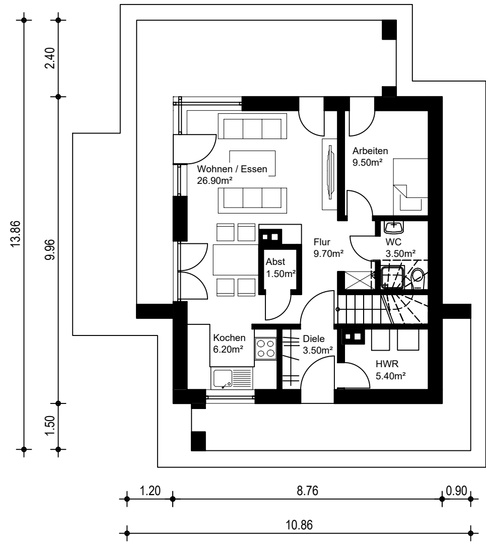
ERDGESCHOSS
