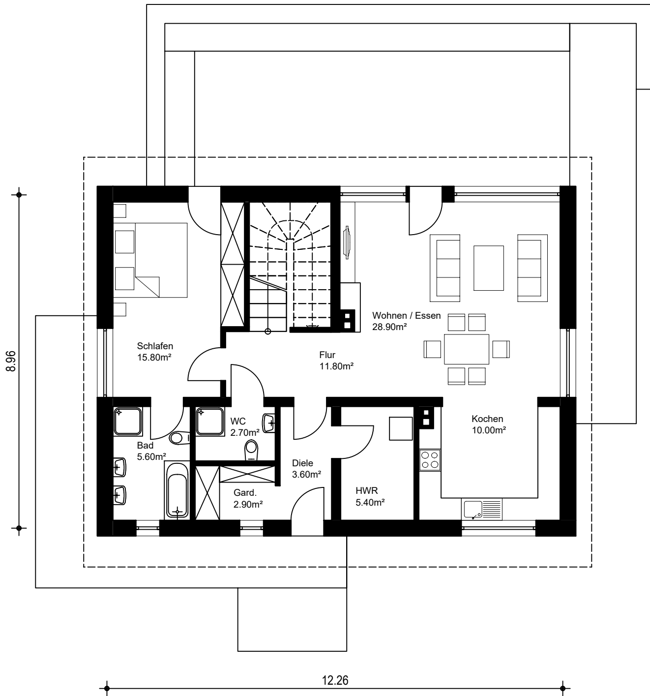
ERDGESCHOSS
