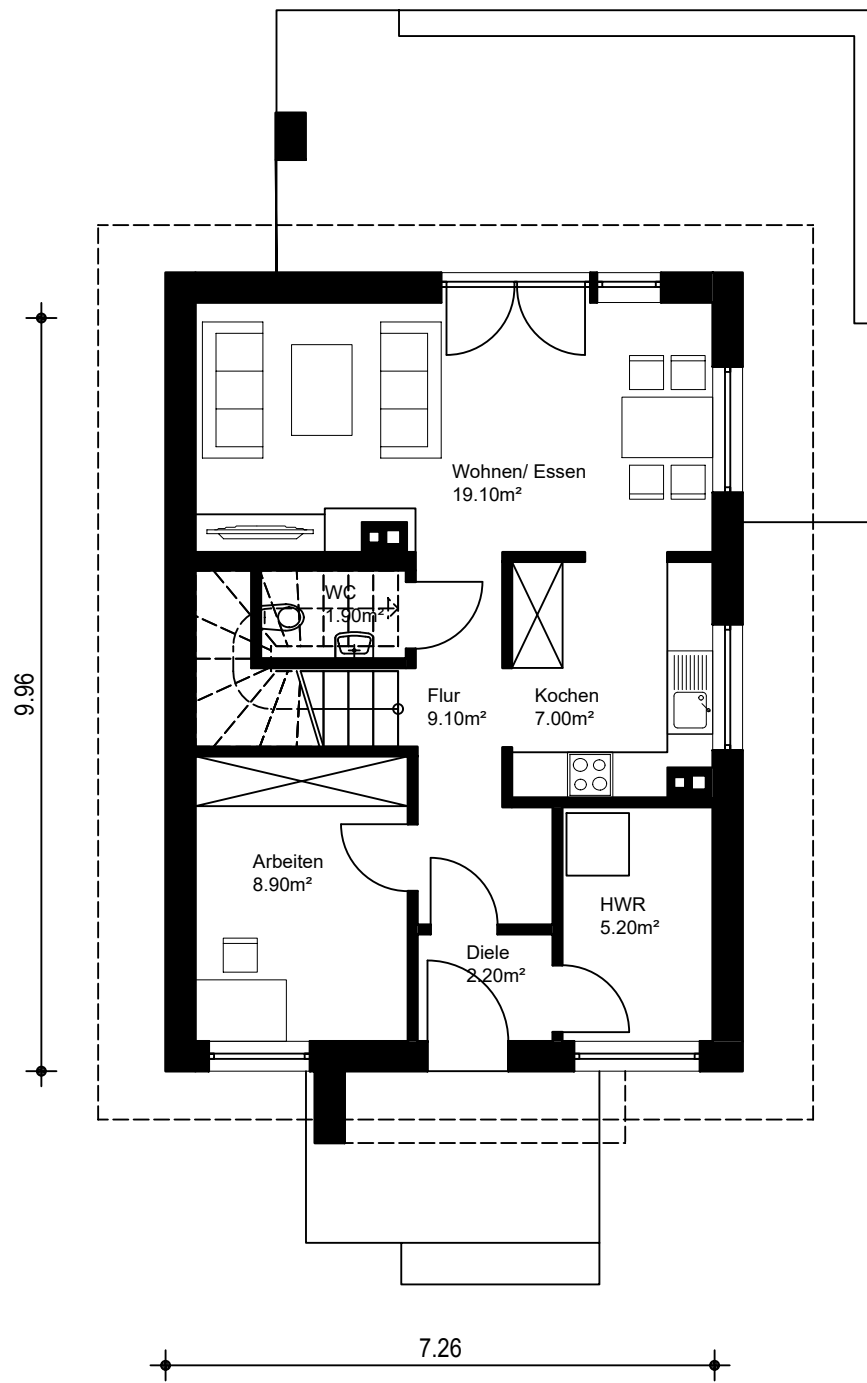
ERDGESCHOSS
